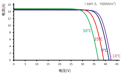
不同电池温度下, I-V 曲线图
